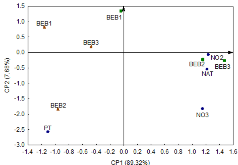
Figura 1 – Gráfico biplot da análise de Componentes Principais (ACP), do córrego São José de Bebedouro (BEB-BEB3) nos períodos de seca e chuva. Pontos azuis representam os parâmetros químicos, NO 3 = Nitrito ( \mu\text{g L}^{-1} ); NO 2 = Nitrito ( \mu\text{g L}^{-1} ); NAT= Nitrogênio Amoniacal Total ( \mu\text{g L}^{-1} ); PT = Fósforo Total ( \mu\text{g L}^{-1} ). Quadrados verdes (Período de Chuva), triângulos marrons (Período de seca)
